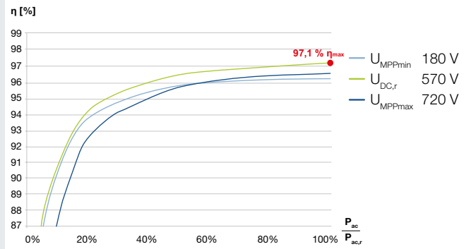
PLENTICORE plus 4.2
